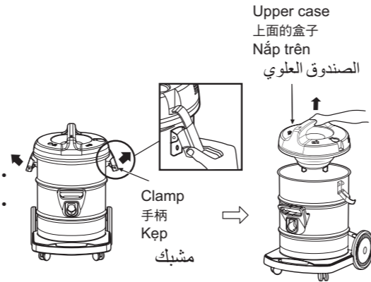
Figure shown is a vacuum cleaner Model CV-960F 此圖為真空吸塵器型號 CV-960F 的圖示 Hình minh hoạ là máy hút bụi kiểu CV-960F الشكل الموضح يمثل الموديل CV-960F من المكنسة الكهربائية
